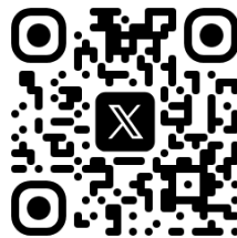
公式 X
